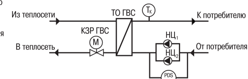
Рисунок 2.2 – Схема контура «ГВС»
