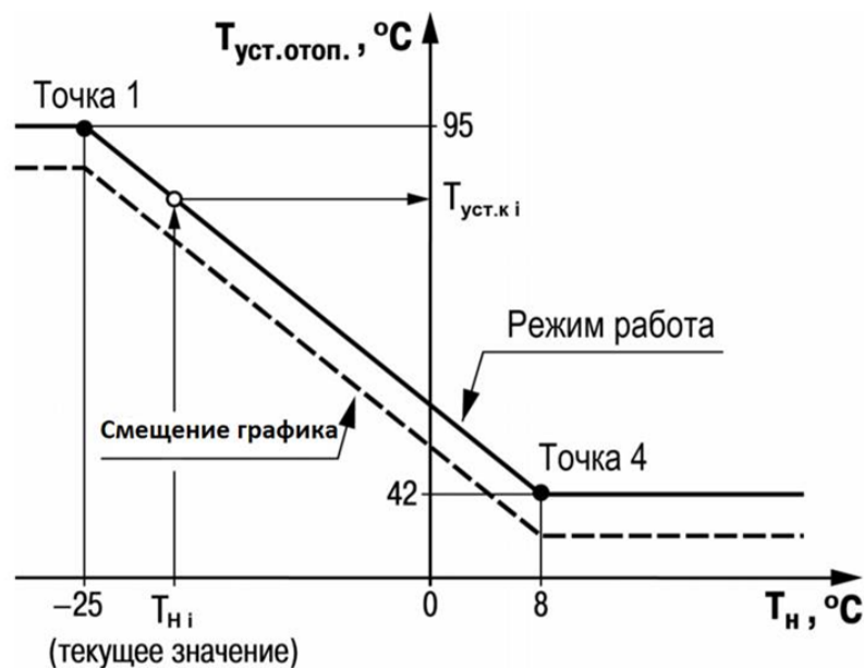
Рисунок 10.3 – Отопительный график
