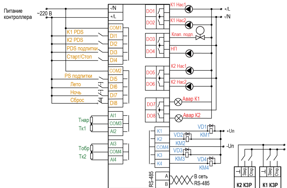
Рисунок 6.3 – Схема подключения
